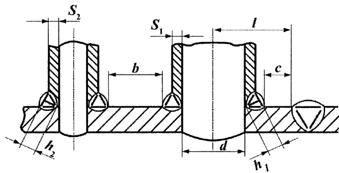
Рис. 10. Расположение сварных соединений приварки патрубков: c \geq 3h_1 ; c \geq 3S_1 ; l \geq 0,9d ; b \geq 3h_2 ; b \geq 3S_2 ( S_2 > S_1 , h_2 > h_1 )
